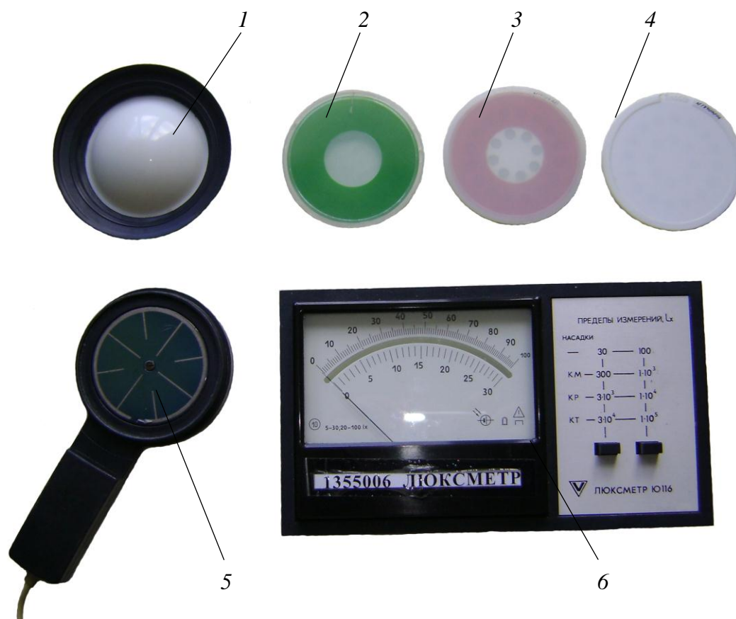
Рис. 2.3. Общий вид люксметра Ю-116:
